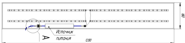
Рис.1 Светильник Офис Тендер 2х36
