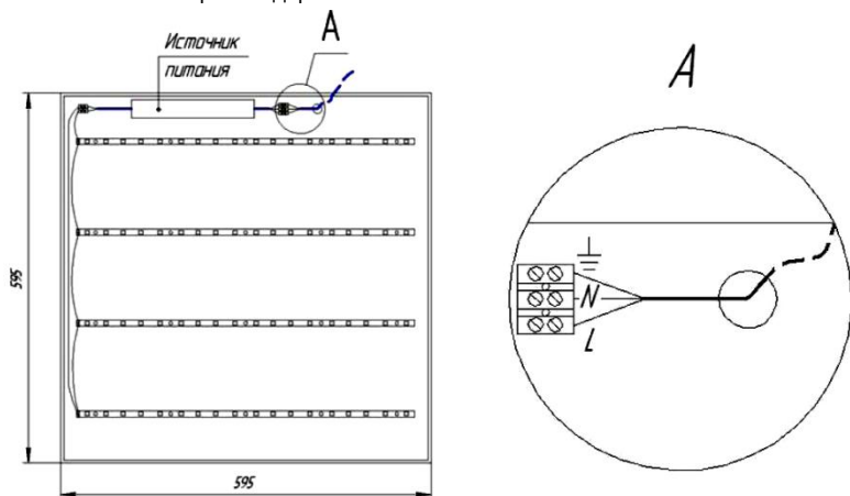
Рис.2 Светильник Офис Тендер 4х18
